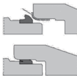
GUARNIZIONE A SCORRIMENTO A CUSPIDE
