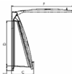
MULTI NB applicazione standard a muro DN 700 – 1500mm
